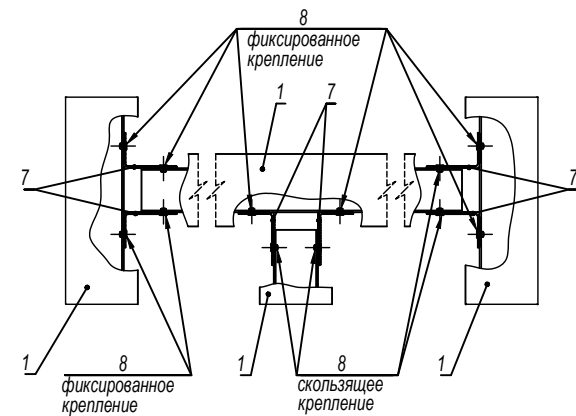
Схема крепления горизонтальной П-направляющей к вертикальным (поз.1) при помощи L-профиля (поз.7)
