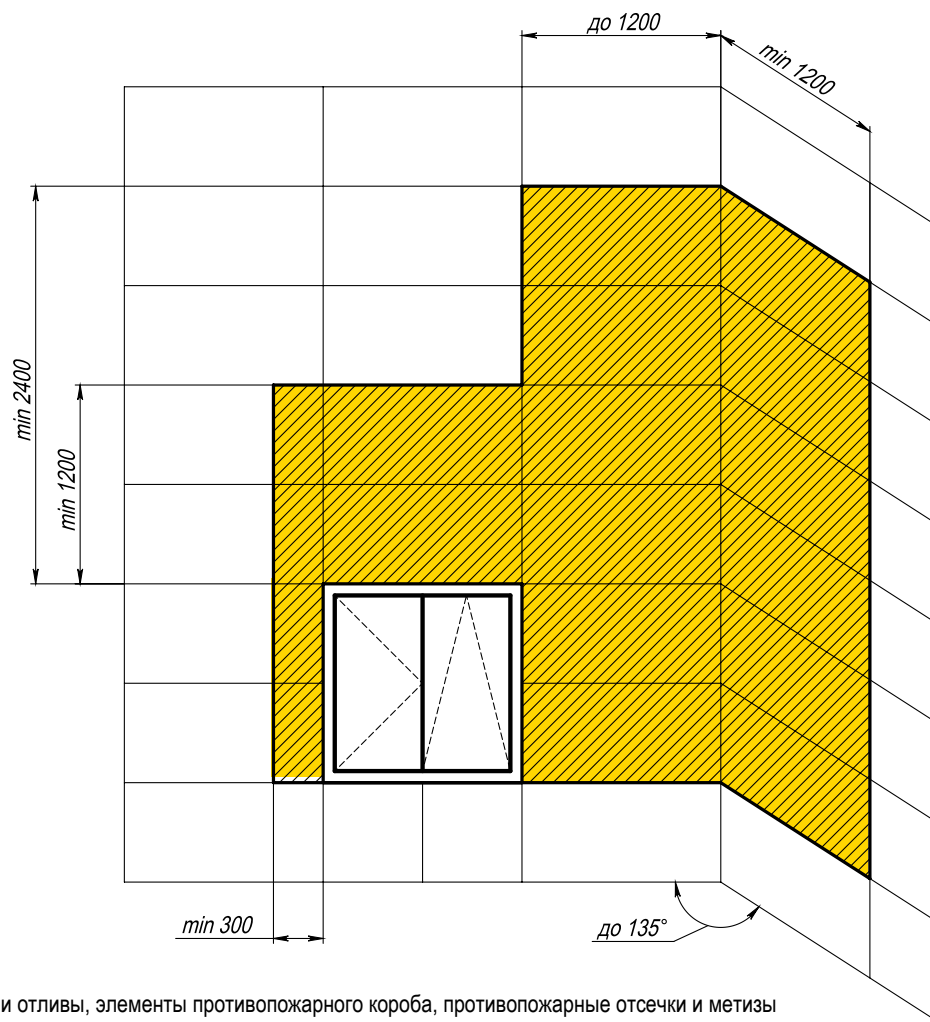
Фрагмент зоны повышенной пожарной опасности с внутренним углом 135 и менее и проемом на расстоянии менее 1,2 м от угла
